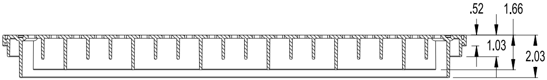
SECTION A-A
